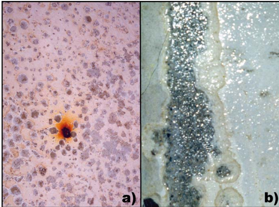
Abbildung 2: Schädigung des Tragwerksbetons a) Bodenfläche eines geschädigten Behälters b) Detailaufnahme eines Fleckens nach der Reinigung
