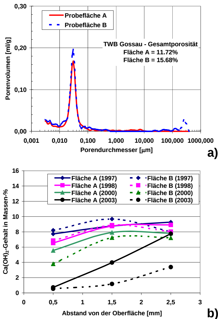
Abbildung 8: a) Mittlere Gesamtporosität und Porengrößenverteilung für Proben aus der Fläche A und B b) Mittlerer Calciumhydroxidgehalt als Funktion der Versuchsdauer für die Fläche A und B
