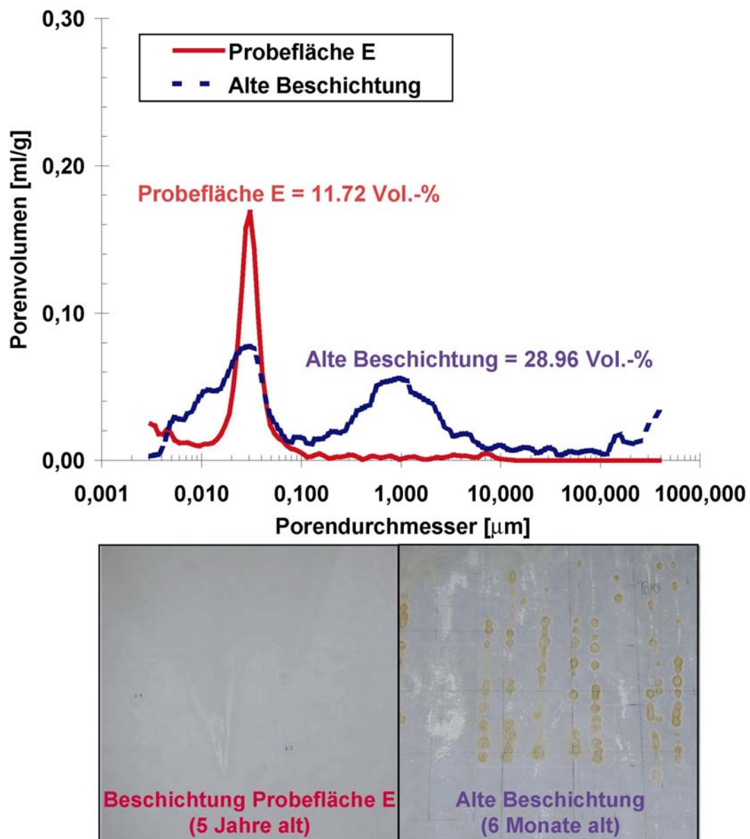
Abbildung 6: Vergleich der Porenkennwerte zwischen den Proben aus der Probenfläche A und Proben einer alten Beschichtung
