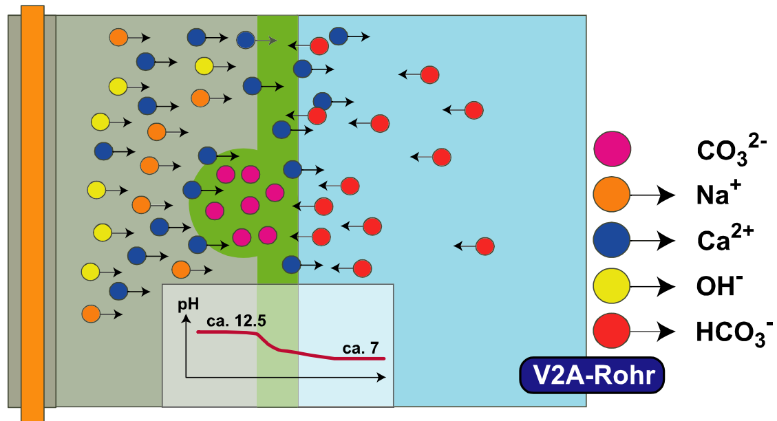
Abbildung 5: Schematische Darstellung der hydrolithischen Korrosion zementgebundener Werkstoffe
