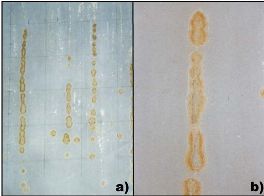
Abbildung 1: Typisches Schadensbild aus einem Trinkwasserbehälter a) Vertikale Anordnung der Flecken b) Zu einem späteren Zeitpunkt wachsen einzelne Flecken zusammen
